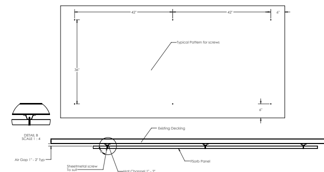
Hat Channel
